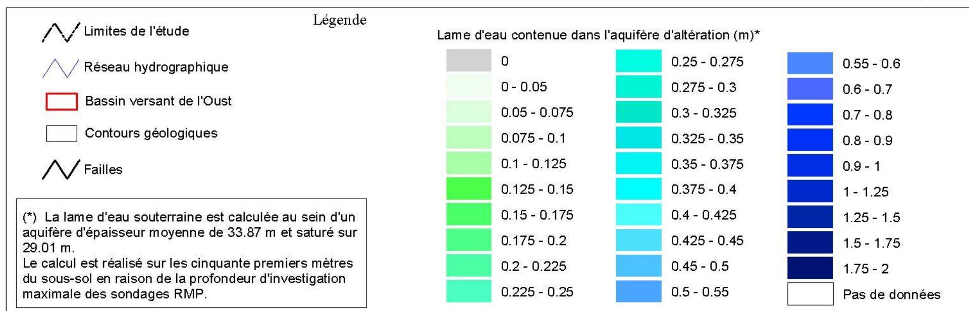
Planche 48 - Lame d'eau totale de l'aquifère d'altération (bassin de l'Oust)
