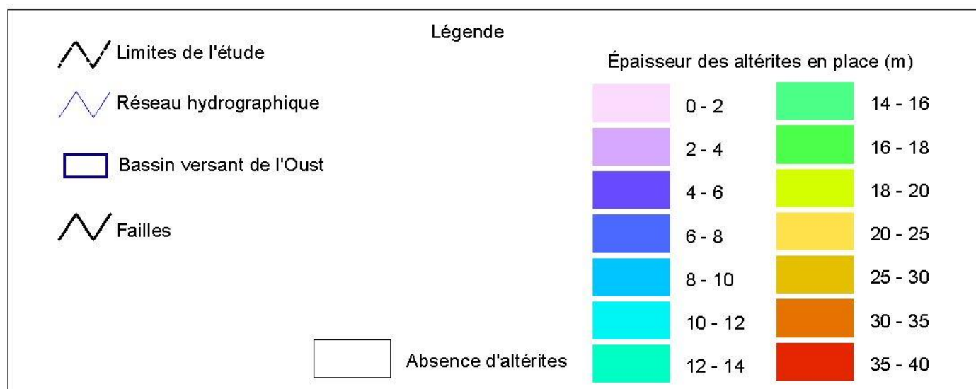
Planche 24 - Épaisseur des altérites en place (bassin de l'Oust)
