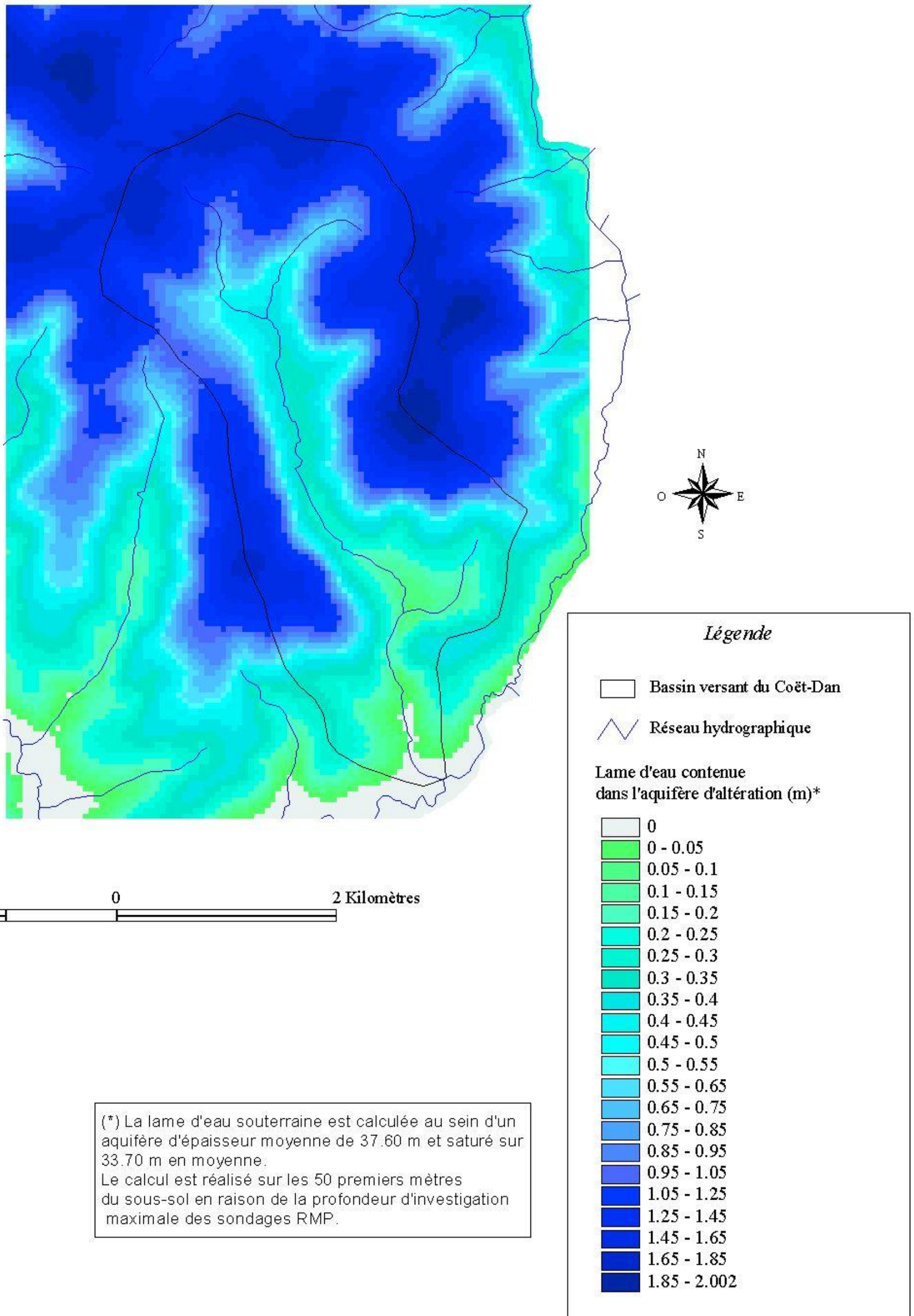
Pl. 36 - Lame d'eau totale de l'aquifère d'altération (bassin du Coët Dan)
