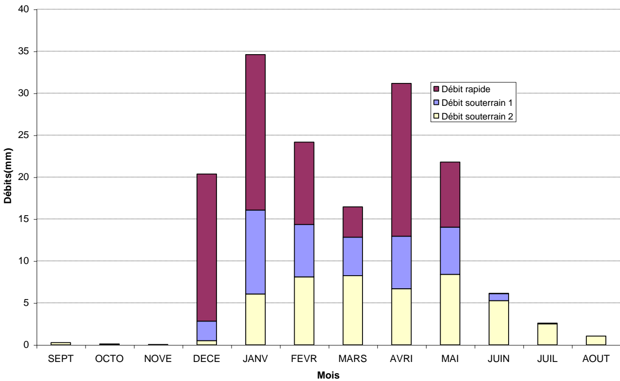
Fig. 21 - Débits mensuels moyens interannuels des bassins versants
