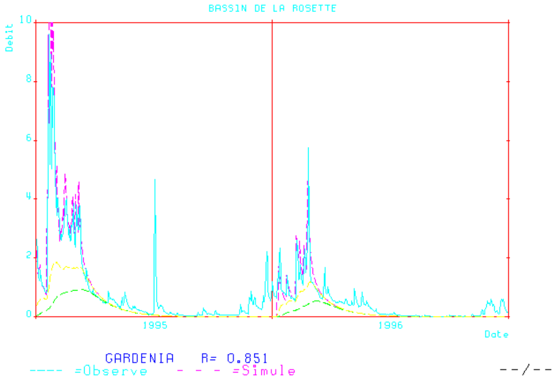
Fig. 18 - Modélisation Gardénia - Calage des paramètres des bassins versants
