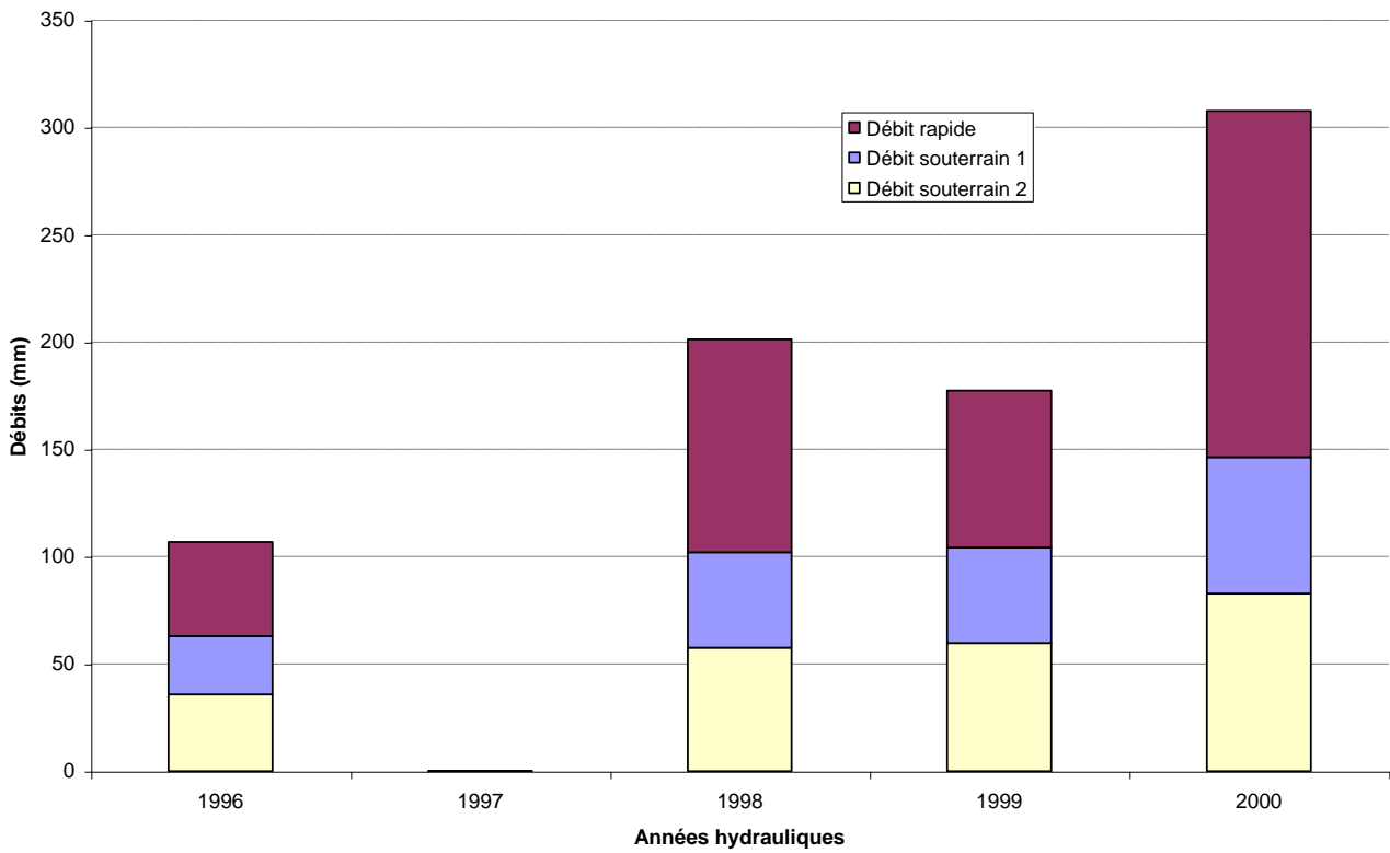
Fig. 20 - Débits annuels rapides et souterrains des bassins versants
