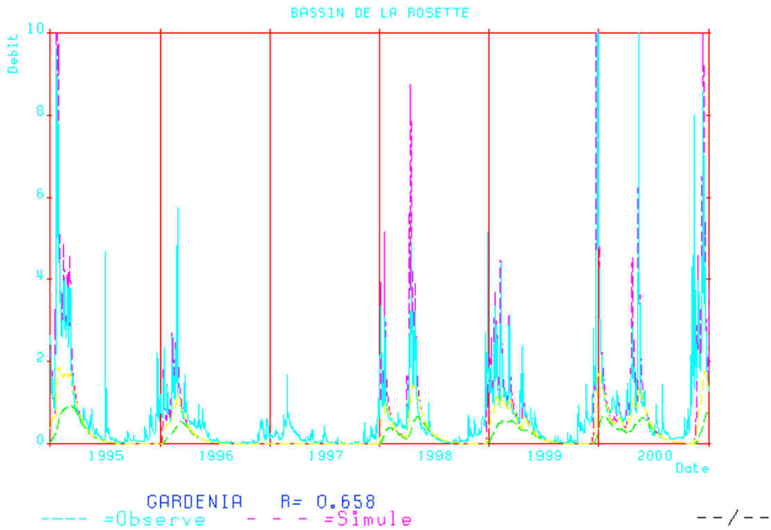
Fig. 19 - Modélisation Gardénia Débits mesurés et calculés des bassins versants
